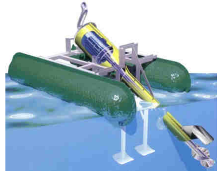
Montage sur flotteurs
